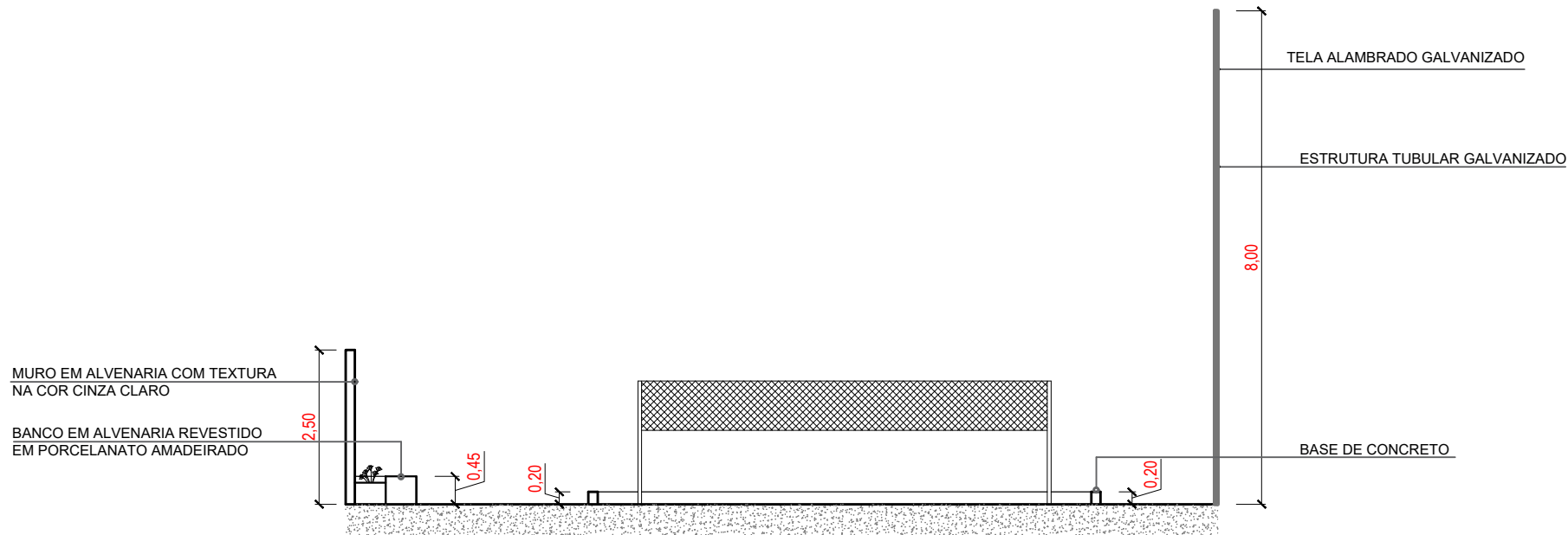
CORTE EE ESCALA_1/75
