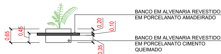
ELEVAÇÃO LATERAL | BANCO 03 ESCALA_1/75
